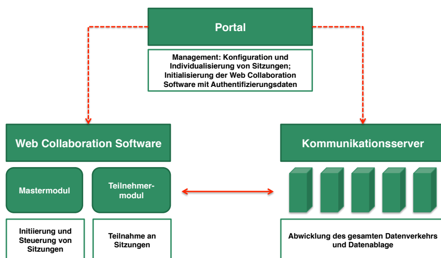
Abb. 4: Architektur von FastViewer
